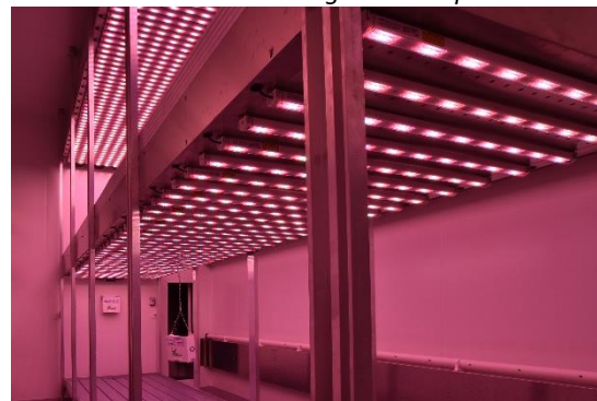
Belichtingsinstallatie voor meerlagenteelt
